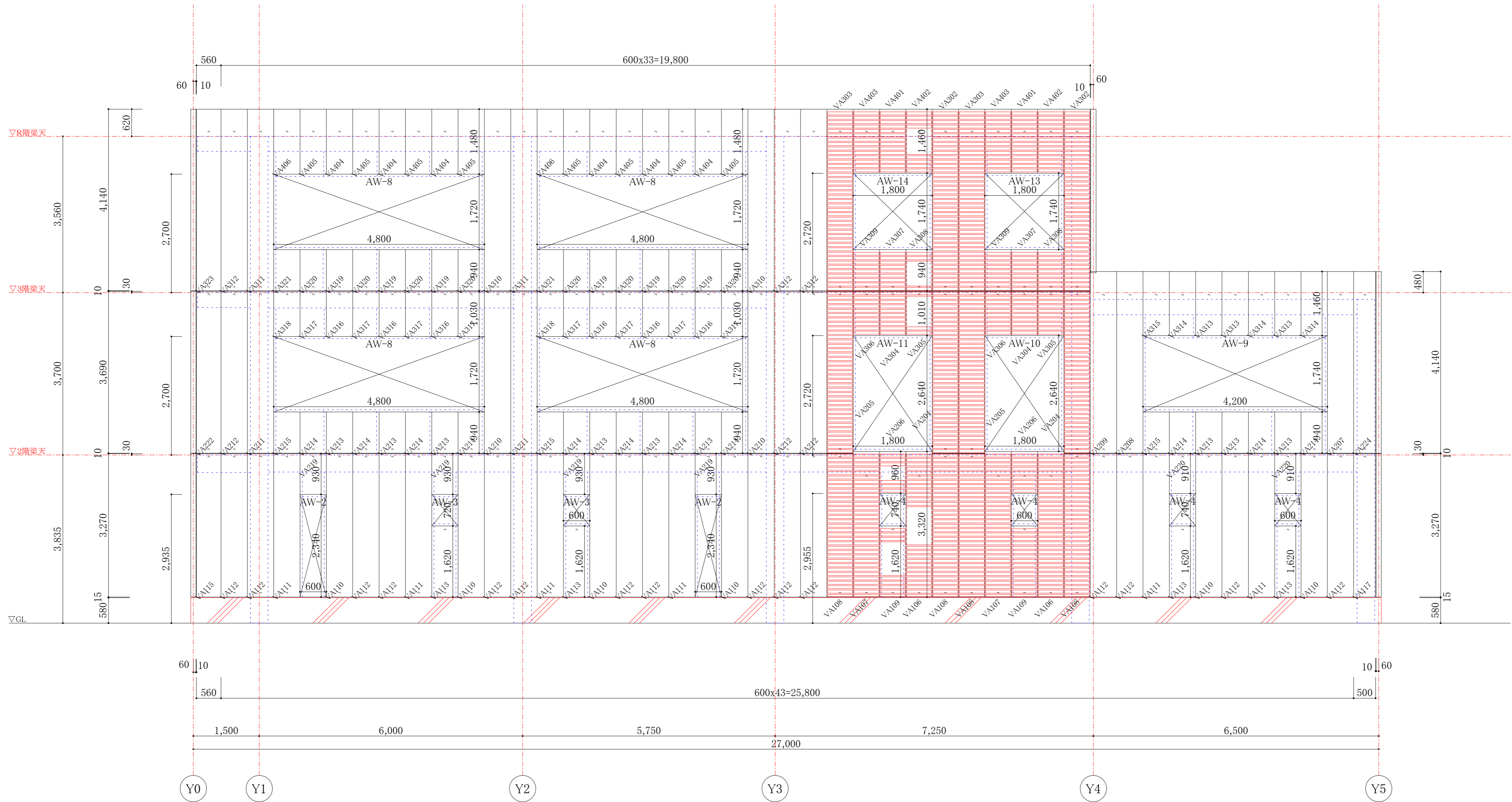
X3通り立面割付図:S=1/60 外壁厚 120
