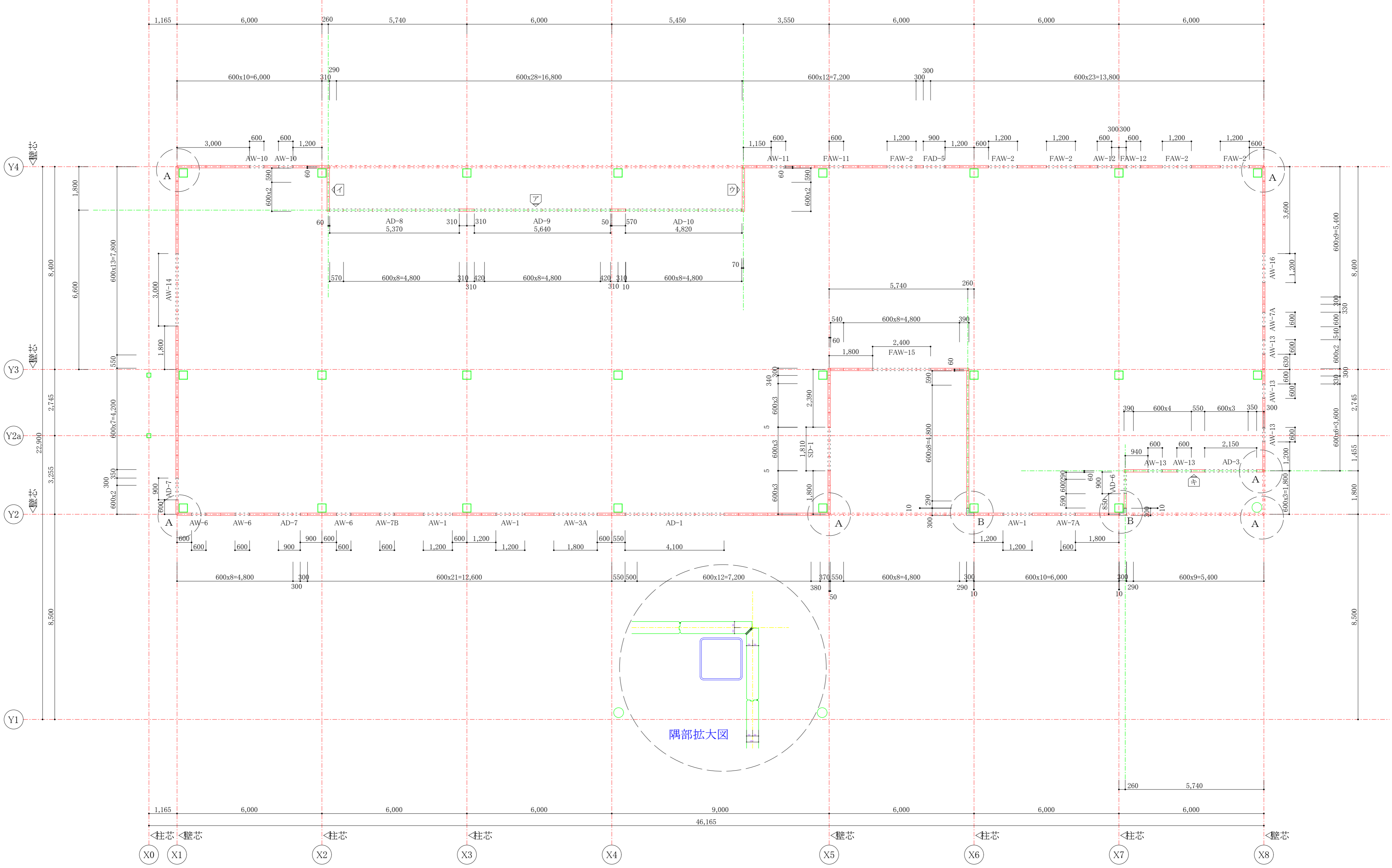
1階平面図:S=1/100
